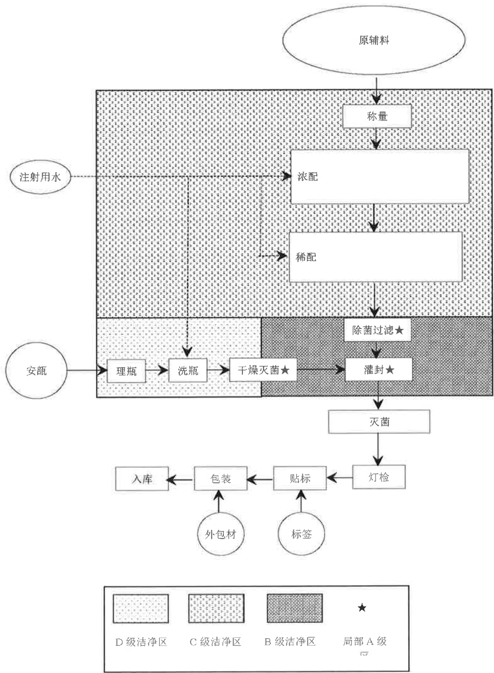
羟喜树碱注射液生产工艺流程图
